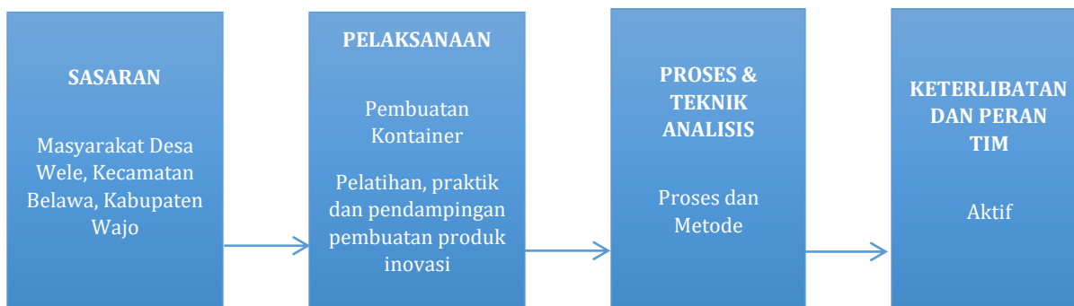
Gambar 1. Alur Kegiatan
